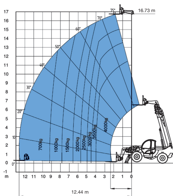
Diagramma di carico (con stabilizzatori)
